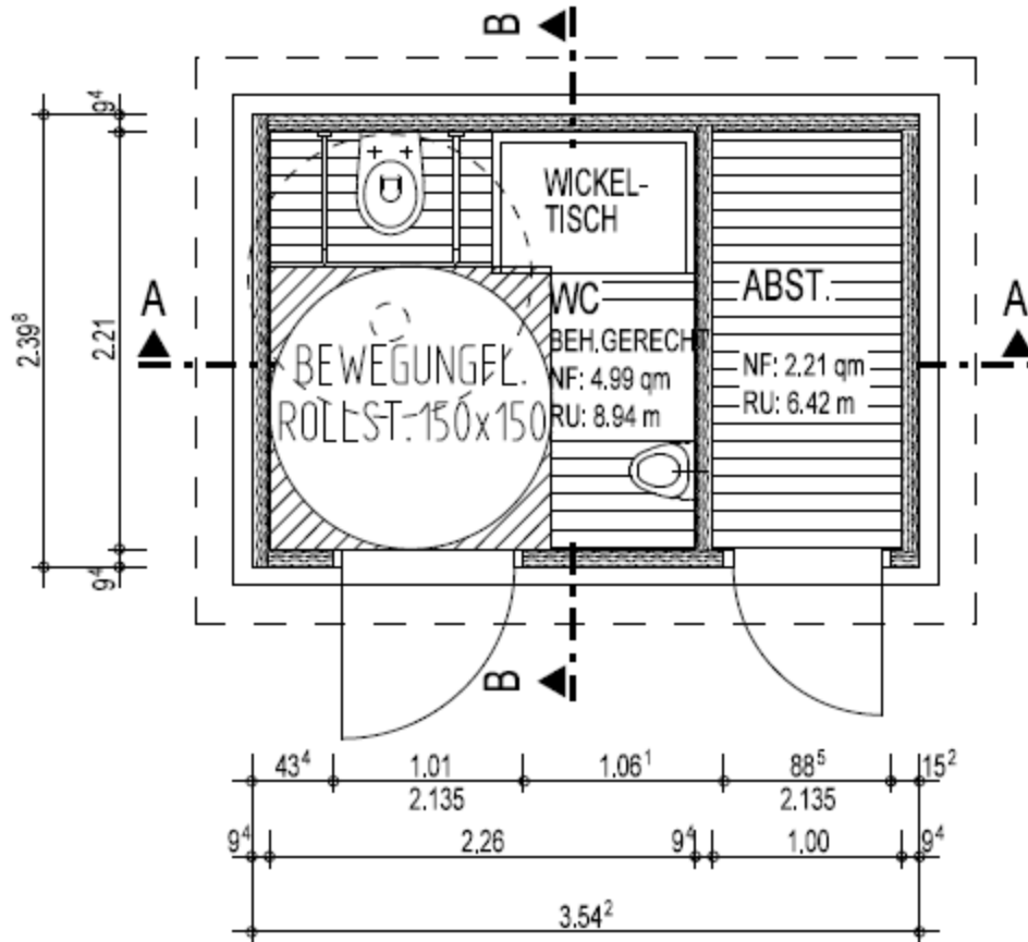
GRUNDRISS
