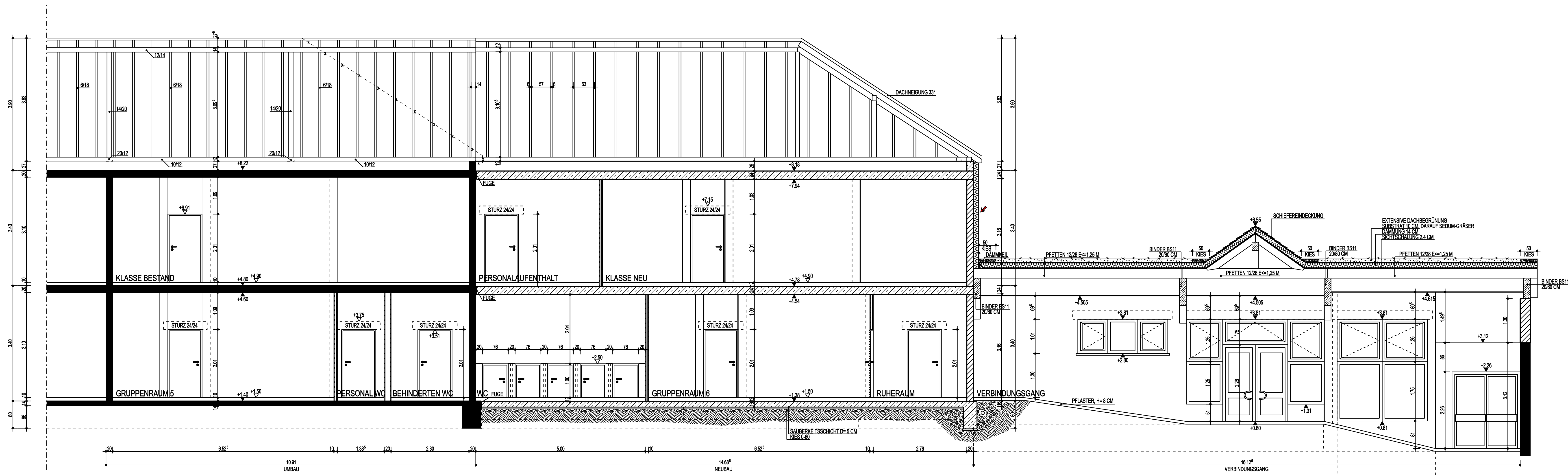
SCHNITT D-D
