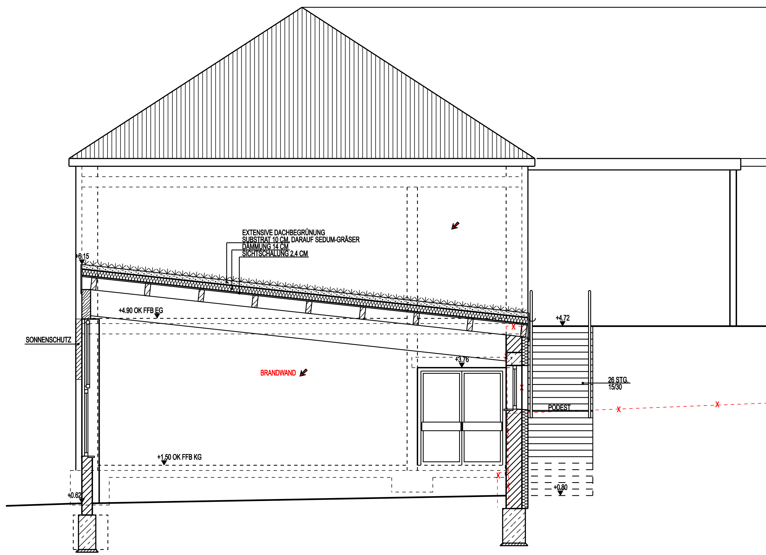
SCHNITT A-A
