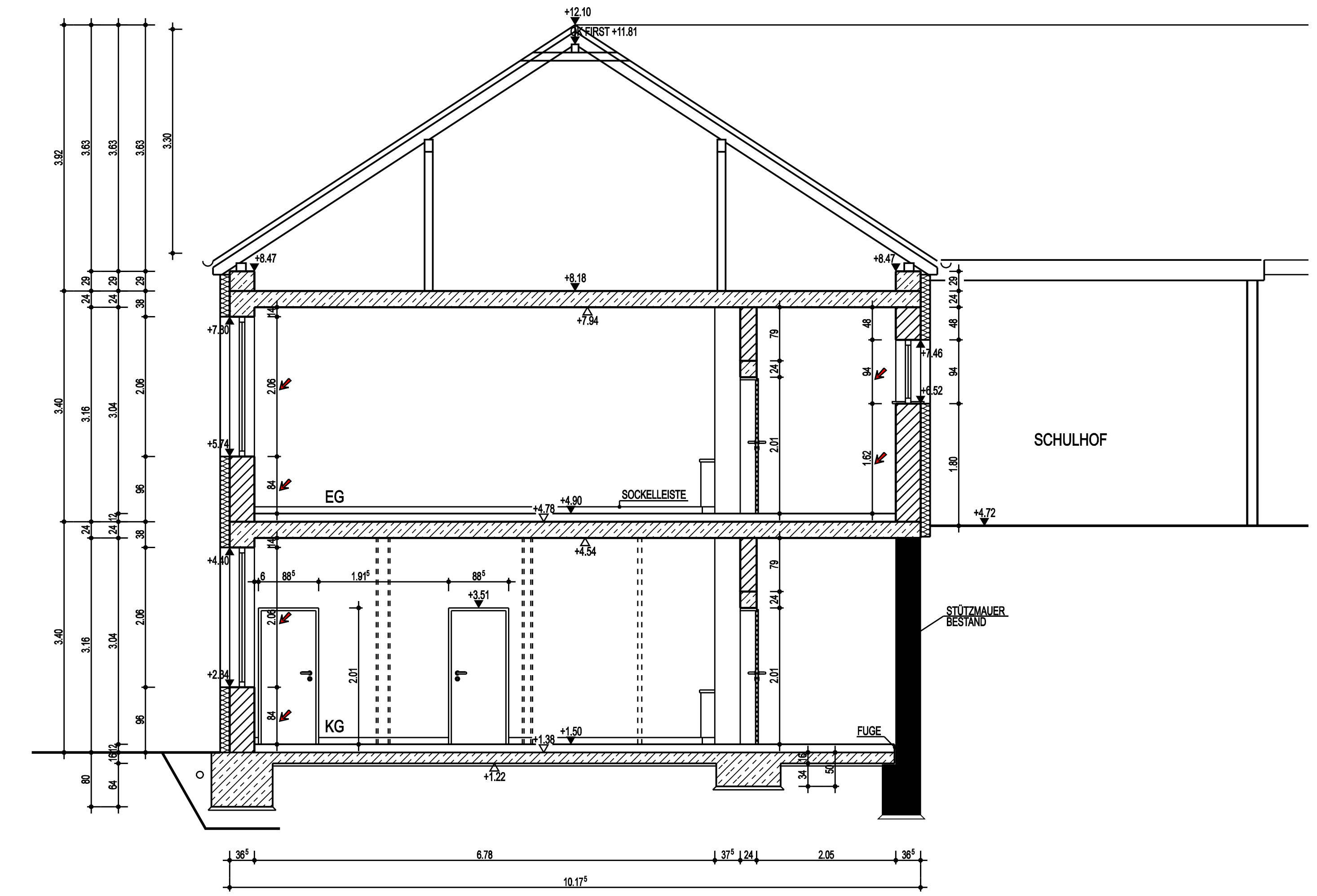
SCHNITT C-C
