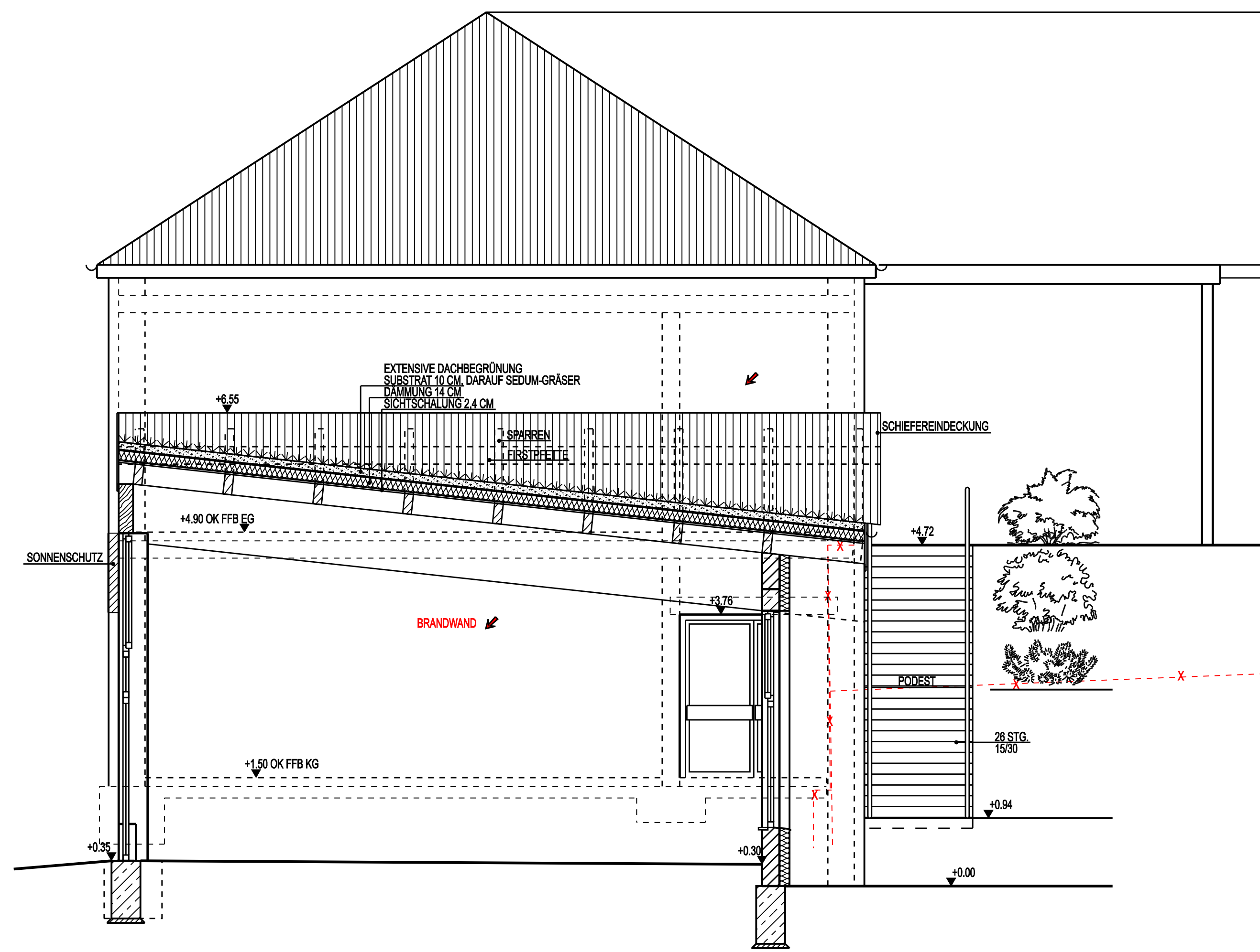
SCHNITT B-B
